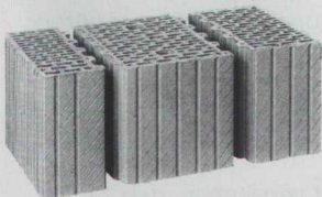
SM 91/SM78 / SM 32 Wanddicke 30,0 cm
