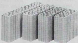
K93/K90/K91/034 Wanddicke 11,5 u. 10,0 cm
