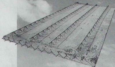
Fertigteil-Decke
