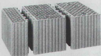
SM 90/ SM74 / SM 15 Wanddicke 36,5 cm
